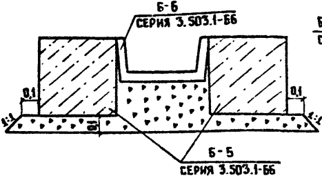
М1:20 2-2
